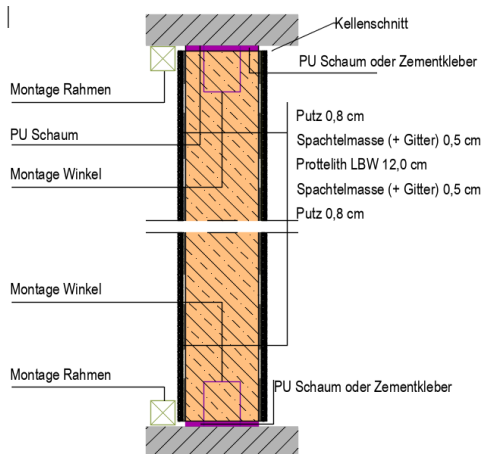
Skizze 1: Decken- und Bodenanschluß
